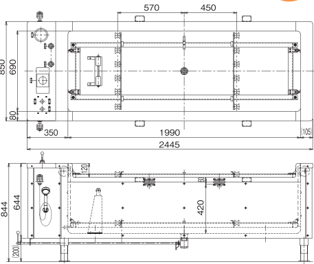
外観図
